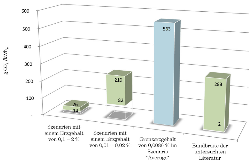
CO 2 Emissionen der nuklearen Brennstoffkette (Wallner et al. 2011)
